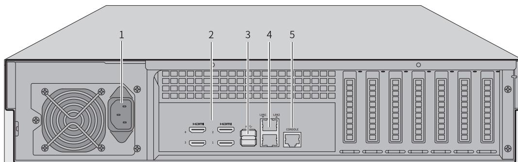
图1-3 TL-TUMS2700-YQ后面板示意图
