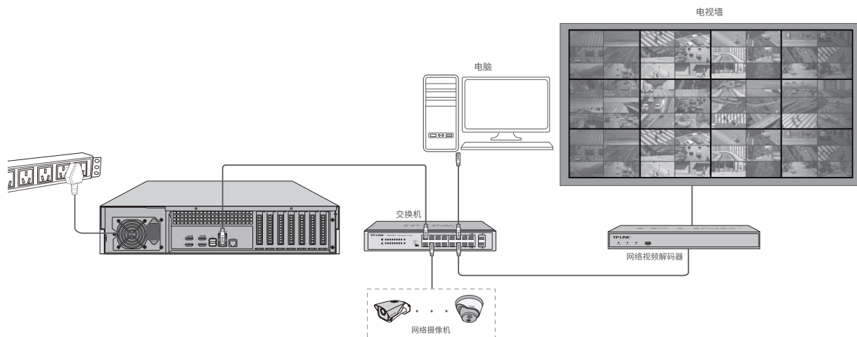
图3-3 设备连接示意图
